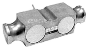
Рисунок 9 - Общий вид датчиков семейства Dual shear beam серии B9E
