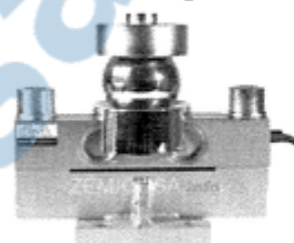
Рисунок 14 - Общий вид датчиков семейства Dual shear beam серии HM9B
